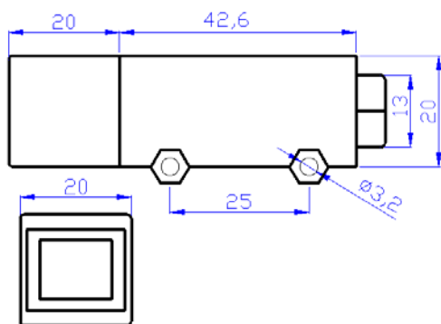
安装尺寸和接线图
